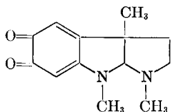
Rubeserine
