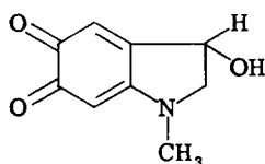
Adrenochrome
