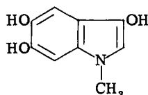
Adrenolutin
